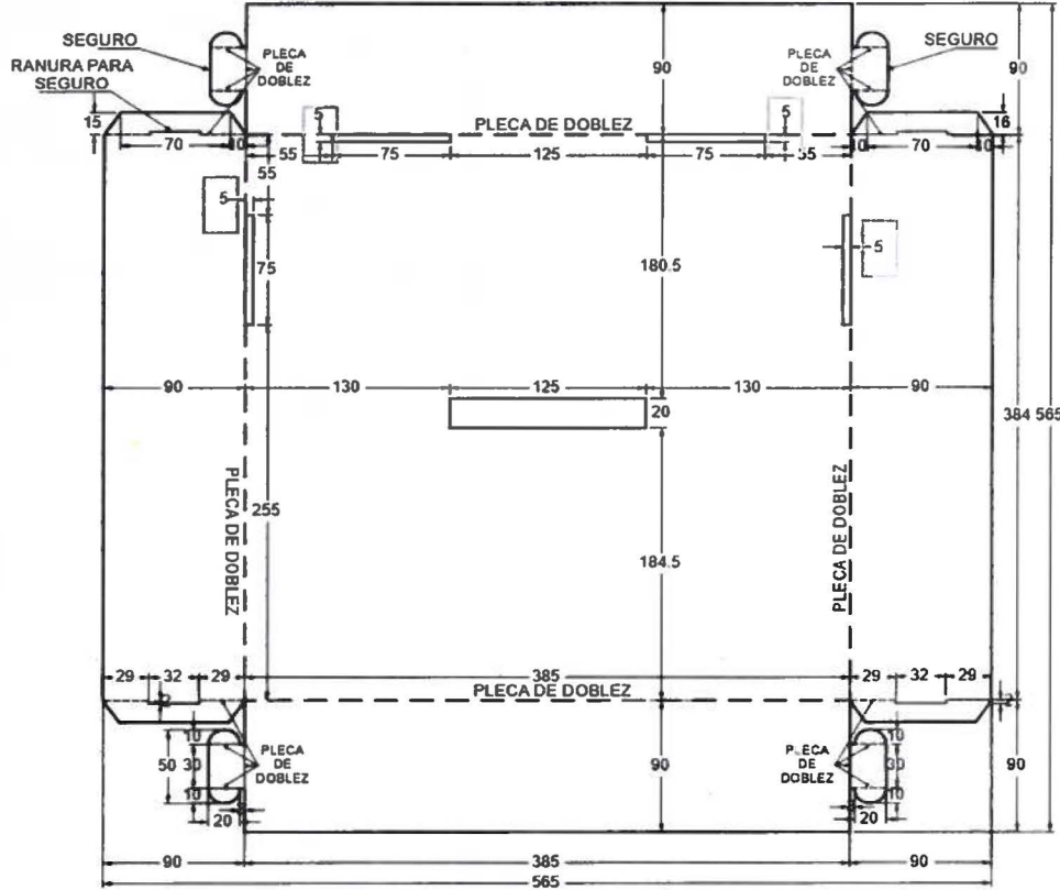
Dimensiones del desarrollo del forro para producción.
