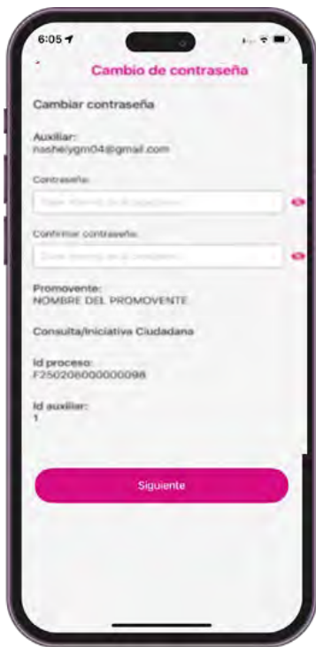
Figura 4.6.5. Captura contraseña.
