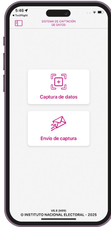
Figura 4.2.22. Menú principal
