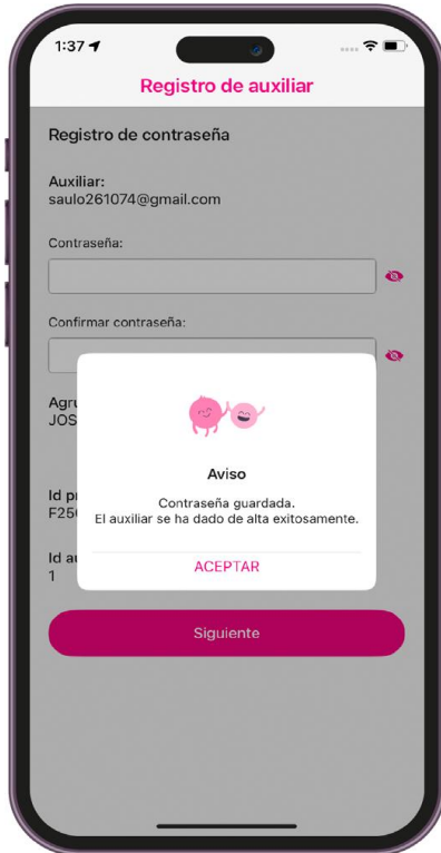
Figura 4.2.21. Contraseña guardada.
