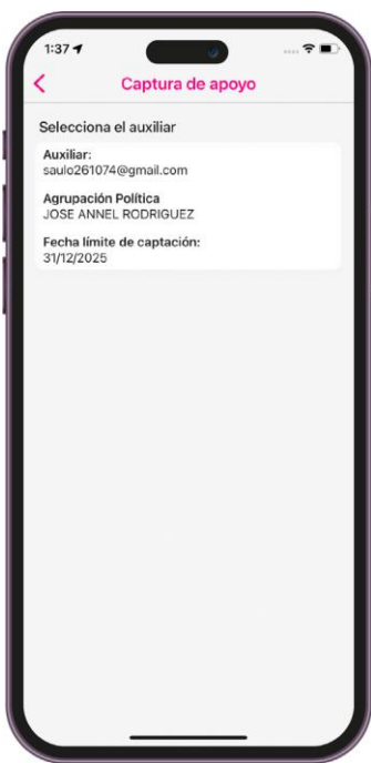
Figura 4.3.2. Auxiliar registrado.
