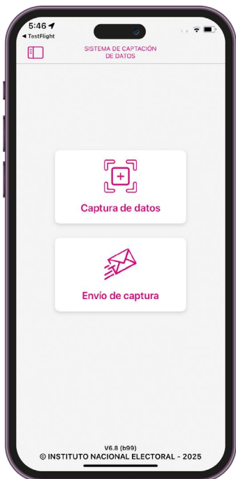
Figura 4.1.6. Menú principal
